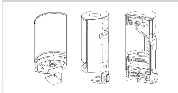
RACCORDEMENT AIR EXTÉRIEUR
