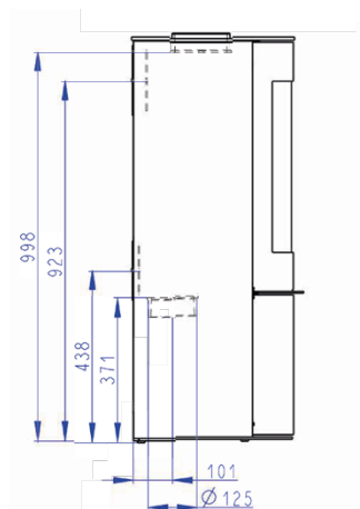
Vue arrière
