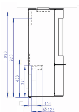
Vue arrière
